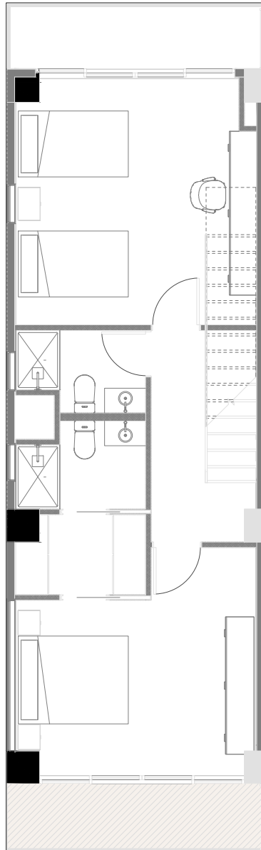
2 | Planta Arquitectonica Nivel 5
