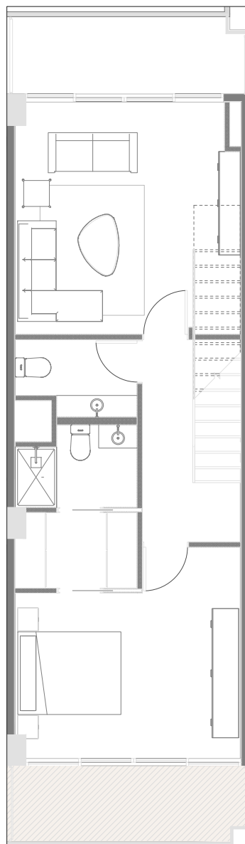
2 | Planta Arquitectonica Nivel 3
