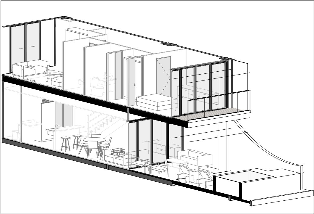
4 | DETALLE NIVEL 1
