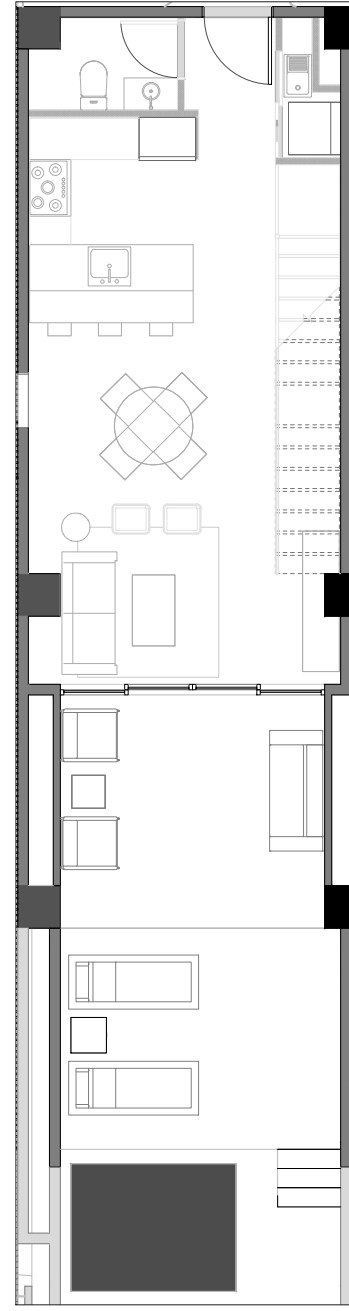
1 | PLANTA ARQ. NIVEL 1
